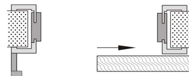
Schiebetür nach rechts öffnend, Konstruktionsprinzip
