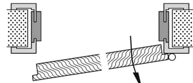
Rechts-drehende Tür, Konstruktionsprinzip
