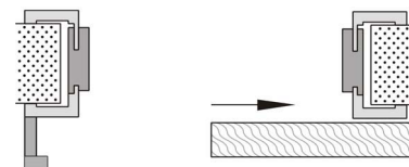
Schiebetür nach rechts öffnend, Konstruktionsprinzip
