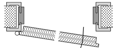
Links-drehende Tür, Konstruktionsprinzip
