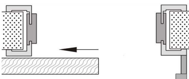
Schiebetür nach links öffnend, Konstruktionsprinzip
